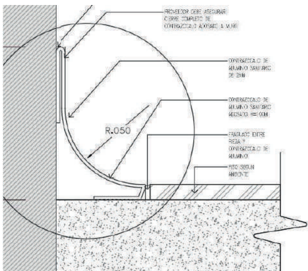
CODIGO: 600607 COLOR: ACERO MATE MEDIDA: 2MM DE ESPEJOR X 10CM DE ALTURA X 2.40MT X TIRA (MODELO # 01)
