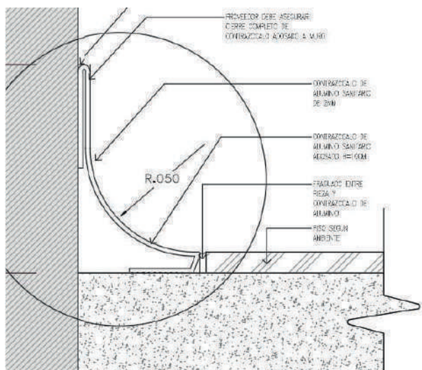
CODIGO: 600605 COLOR: ALUMINIO MATE MEDIDA: 2MM DE ESPEJOR X 10CM DE ALTURA X 2.40MT X TIRA (MODELO # 01)
