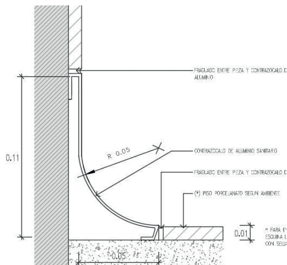
CODIGO: 600606 COLOR: ALUMINIO MATE MEDIDA: 2MM DE ESPEJOR X 10CM DE ALTURA X 2.40MT X TIRA (MODELO # 02)
